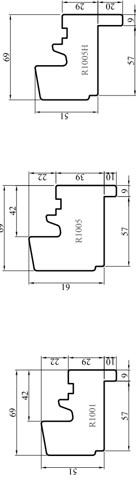
Appui rénovation
