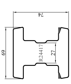
Ouvrant 74 rainure de 47
