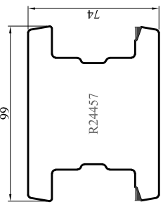
Traverse intermédiaire ouvrante
